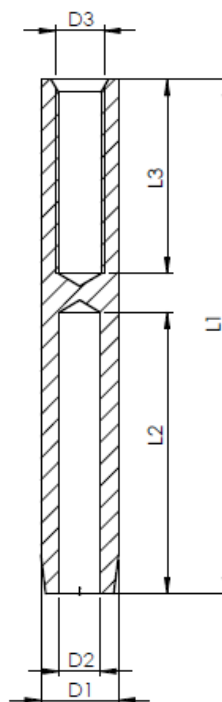
SCHNITT A-A
